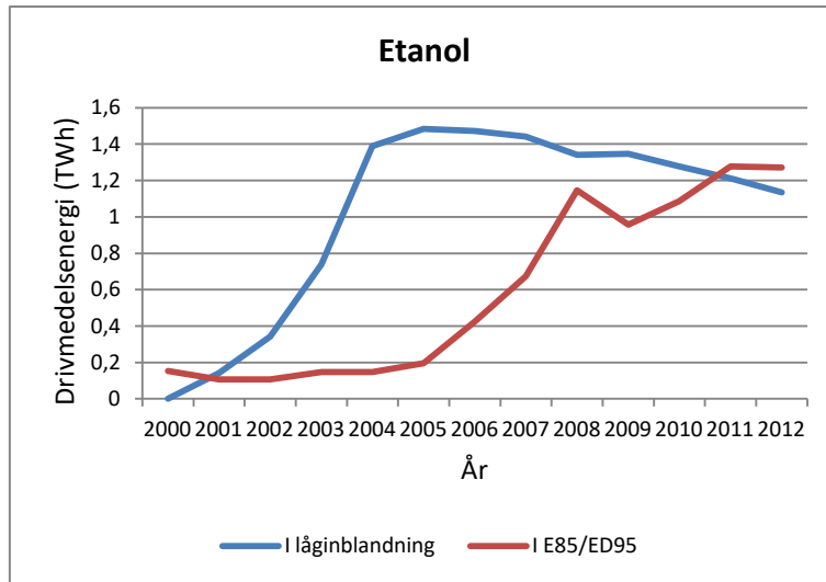
Figur 4.5 Den energimängd ren etanol som levererats i Sverige per år, uppdelad i etanol som låginblandats i bensin, och etanol som säljs i drivmedelskvaliteter där etanolen är huvudingrediens ED95 innehåller 95 % etanol och används i anpassade dieselmotorer, främst i tyngre fordon som bussar. (Källor: Energimyndigheten och SCB)
